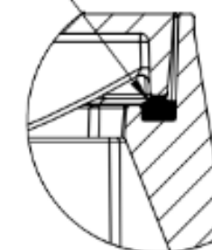
EPDM tesnilo
