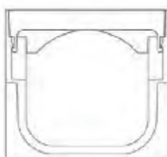
Samopritrdilni sistem za PE-HD rešetke.
