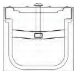
Pritrjevanje z ročico in vijakom za vročje cinkane in LTŽ rešetke. 1 set na kanaletu AbarWDK110
