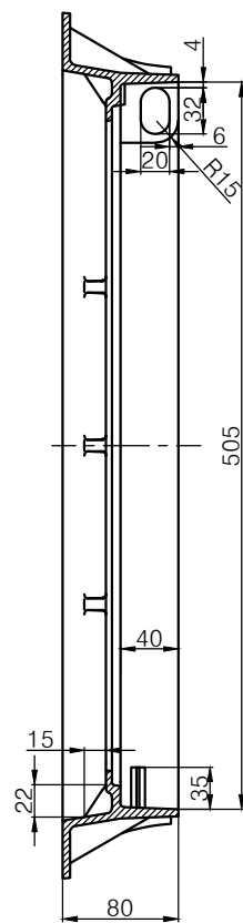
B-B
